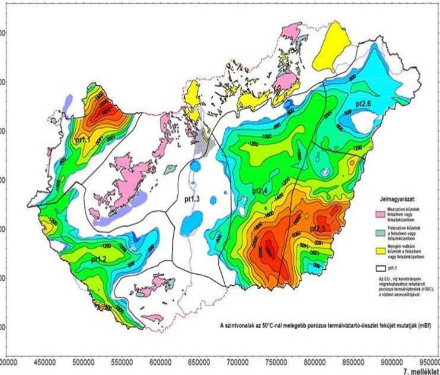
50°C-nál melegebb porózus termálvizadó rétegek elterjedése
